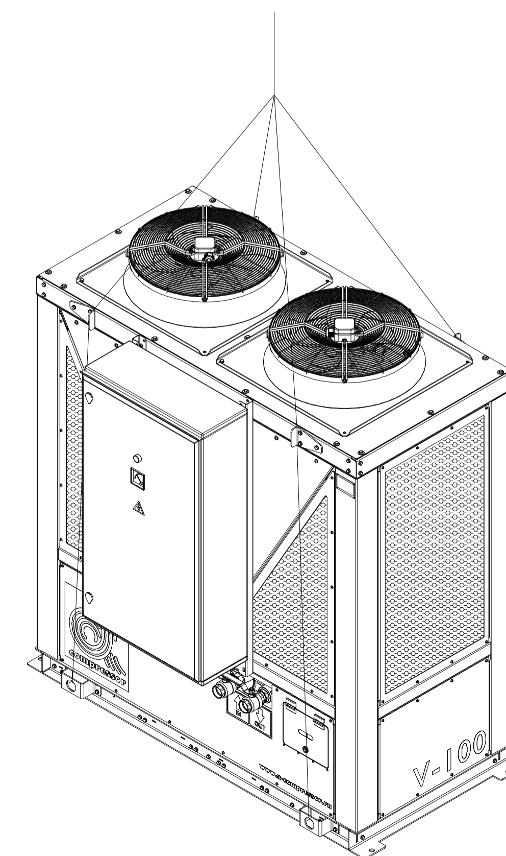
Схема строповки
